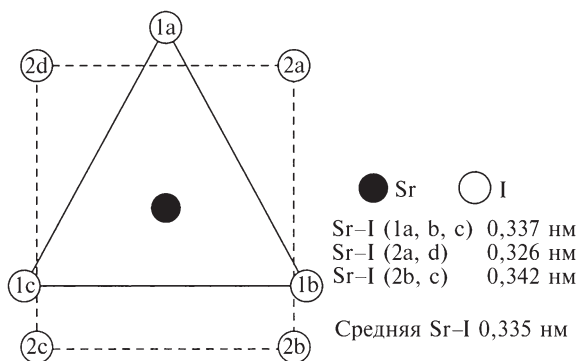
Рис. 5.3. Структура SrI 2 , в которой КЧ Sr равно 7. Плоскости 1 и 2 почти параллельны (4,5°), а плоскости 1a2a2d и 1b2b2c1c находятся под углом 12° друг к другу [9]
