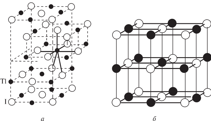
Рис. 7.10. Структура желтого \text{TiI} (а) и ее родство со структурой \text{NaCl} (б). Атом \text{Ti} имеет ближайшее окружение из 5 атомов иода в 5 вершинах октаэдра и 2I + 2Ti во второй координационной сфере. Один атом иода находится на расстоянии 0,336 нм, 4 — на расстоянии 0,349 нм и 2 — на расстоянии 0,387 нм, а одно из двух кратчайших расстояний \text{Ti}-\text{Ti} равно 0,383 нм. Красные формы \text{InX} ( \text{X} = \text{Cl}, \text{Br}, \text{I} ) имеют похожие структуры [43]
