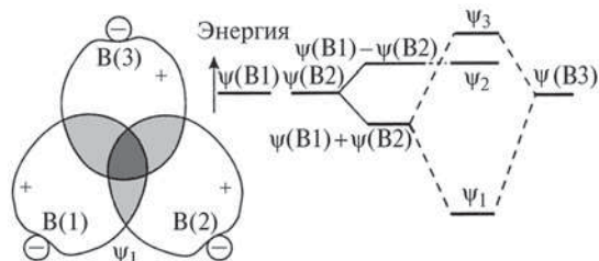
Рис. 6.13. Образование связывающей центральной трехцентровой связи \psi_1 и схематическое изображение энергий трех молекулярных орбиталей \psi_1 , \psi_2 и \psi_3
