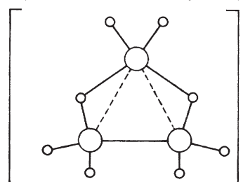
(19) B_3H_8^-
