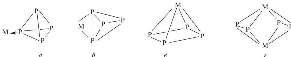
Рис. 12.9. Схематическое изображение различных типов координации: a — \eta^1 - P_4 ; б — \eta^2 - P_4 ; в — \eta^4 - \text{цикло-}P_4 ; г — (\mu, \eta^2-P_2)_2 (см. текст)
