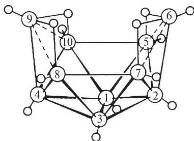
(36) B_{10}H_{14}
