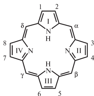
(1) Порфин
