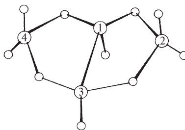
(13) B_4H_{10}
