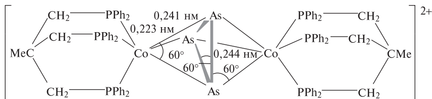
Рис. 13.23. Структура катиона [L^*Co-\mu-(\eta^3-As_3)CoL^*]^{2+}
