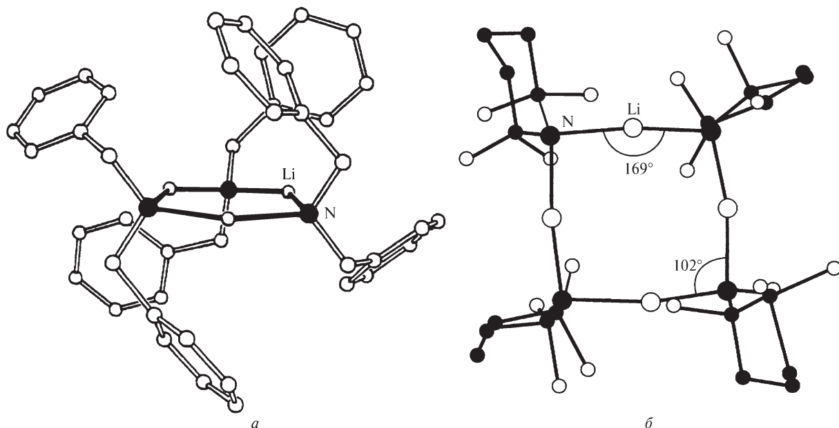
Рис. 4.15. Строение дибензиламилолития [(\text{PhCH}_2)_2\text{NLi}]_3 [81] (а) и тетраметилпиперидинолития [\text{Me}_2\text{C}(\text{CH}_2)_3\text{CMe}_2\text{NLi}]_4 [82] (б) по данным PCA
