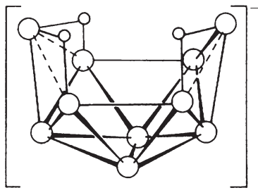
(37) B_{10}H_{13}^-
