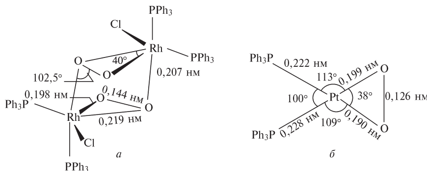
Рис. 14.6. Строение и основные параметры комплексов [(\text{PPh}_3)_2\text{RhCl}(\mu\text{-O}_2)]_2 (а) и [\text{Pt}(\text{O}_2)(\text{PPh}_3)_2] (б). Данные для второго комплекса менее надежны из-за трудности выращивания кристаллов, пригодных для исследования, и их неустойчивости по отношению к рентгеновскому излучению (погрешность измерения длин связи \pm 0,005 нм, погрешность измерения углов \pm 2^\circ )
