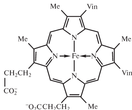
(2) Гем
