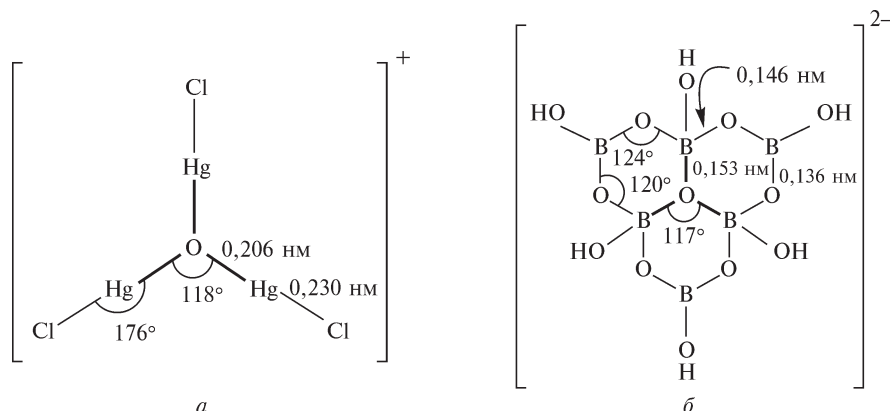
Рис. 14.3. Примеры плоско-треугольного координационного окружения атома кислорода: катион в соединении [O(HgCl)_3]Cl (а) и центральный атом О в дискретном анионе [OB_6O_6(OH)_6]^{2-} в макалестерите (б) — три гетероцикла в одной плоскости, а шесть групп ОН лежат вне плоскости.
