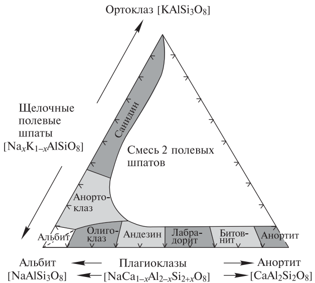
Рис. 9.14. Тройная фазовая диаграмма для полевых шпатов. Точное положение фазовых границ зависит от температуры 3Ca(Al 3 ) 2 Si 2 O 8 анортит (полевой шпат) Ca 3 (Al 6 ) 2 (SiO 4 ) 3 гроссуляр (Ca-гранат)
