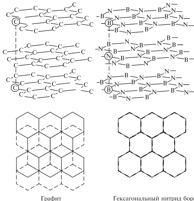
Рис. 6.27. Сравнение гексагональных слоистых структур BN и графита. В BN атомы одного слоя расположены прямо над атомами соседнего слоя, образуя контакты B \cdots N . В графите атомы углерода из одного слоя расположены над пустотами соседнего слоя и прямо над атомами последующего слоя
