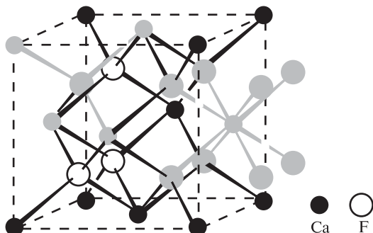
Рис. 5.2. Элементарная ячейка CaF 2 : ионы Ca имеют кубическую координацию 8 ионами фтора, а ионы F — тетраэдрическую координацию 4 ионами кальция. Структуру можно рассматривать как гранецентрированную кубическую решетку из ионов Ca в которой все тетраэдрические пустоты заняты ионами F
