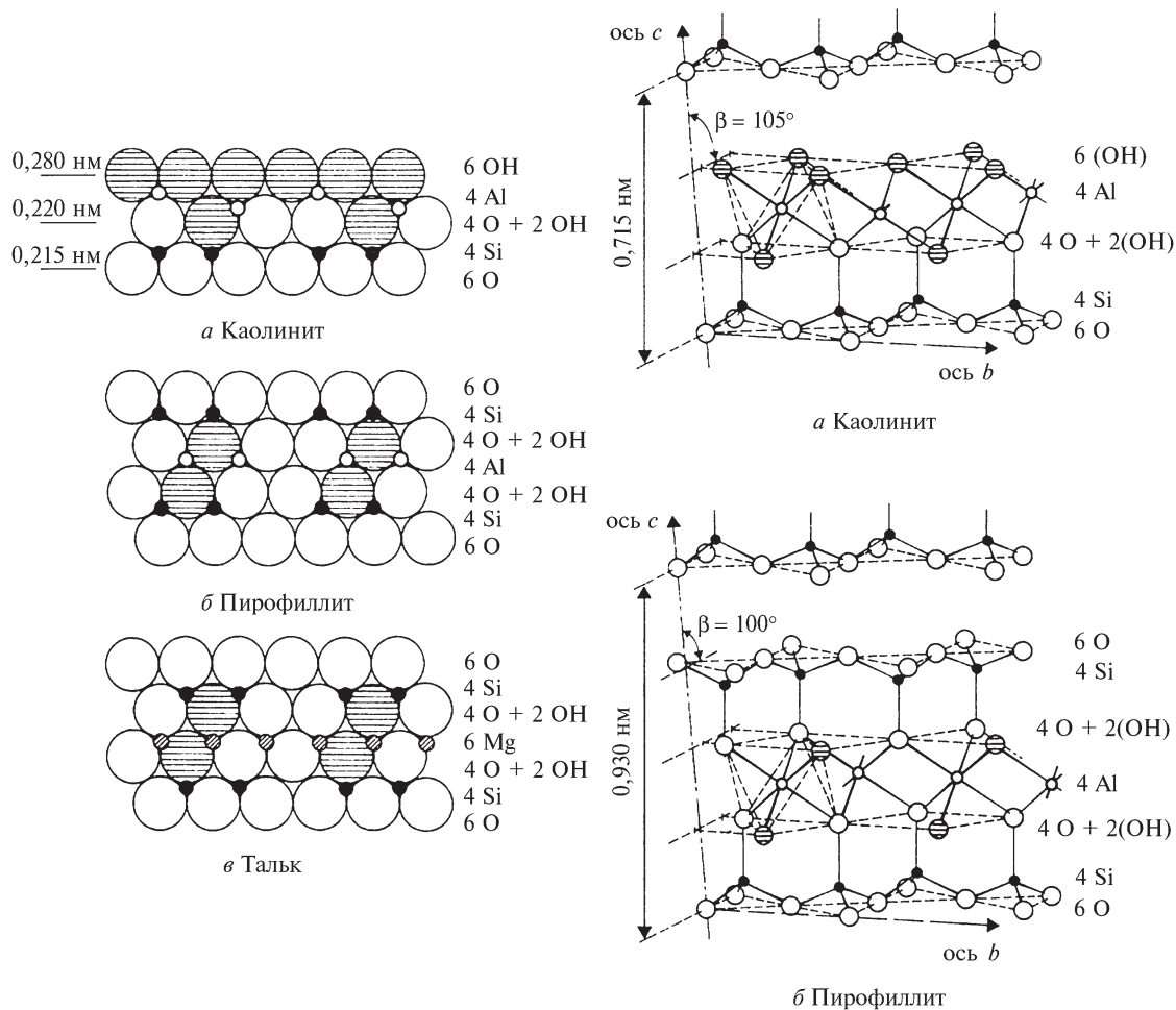
Рис. 9.11. Альтернативные представления слоистых структур: a — каолинит; б — пирофиллит; в — тальк. [Emeléus H.J., Anderson J.S., 1960; Mason B., Berry L.G., 1968]
