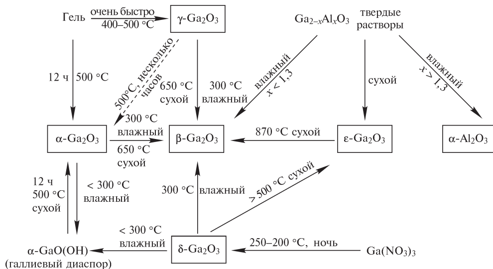
Рис. 7.13. Схема, иллюстрирующая взаимные переходы различных форм оксидов галлия и их гидратов. Переход (во влажном состоянии) фазы, обозначенной как Ga_{2-x}Al_xO_3 , в \beta\text{-Ga}_2O_3 происходит только при x < 1,3 ; если x > 1,3 , образуется структура \alpha\text{-Al}_2O_3
