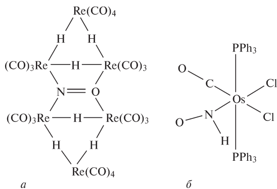
Рис. 11.14. Четверной мостик NO в анионе [\{\text{Re}_3(\mu\text{-H})_3(\text{CO})_{10}\}_2(\mu_4\text{-}\eta^2\text{-NO})]^- ( a ). Нейтральный комплекс [\text{Os}(\text{CO})\text{Cl}_2 \cdot (\text{HNO})(\text{PPh}_3)_2] ( б )
