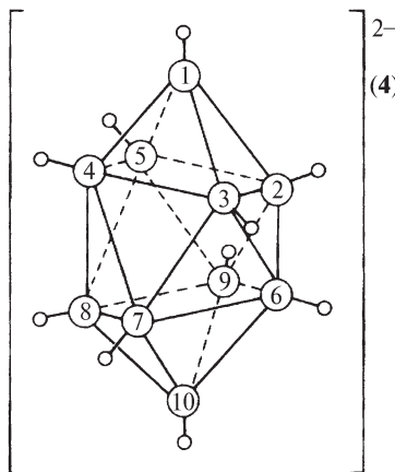
(5) Декагидро-клозо-декаборат(2-) B_{10}H_{10}^{2-}
