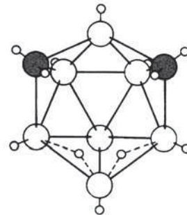
(67) арахно -1,3- C_2B_7H_{13}
