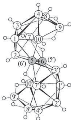
(31) n-B_{18}H_{22} (центросимметричный)
