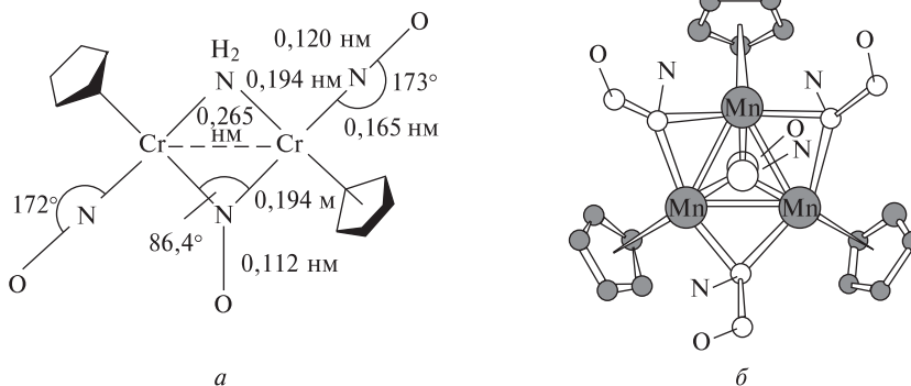
Рис. 11.13. Строение полиядерных нитрозильных комплексов: a — [\{\text{Cr}(\eta^5\text{-C}_5\text{H}_5)(\text{NO})\}_2(\mu\text{-NH}_2)(\mu_2\text{-NO})] с линейной координацией концевой группы NO и двойным мостиком NO; б — [\text{Mn}_3(\eta^5\text{-C}_5\text{H}_5)_3(\mu_2\text{-NO})_3(\mu_3\text{-NO})] с двойными и тройным мостиками NO; молекула имеет симметрию C_{3v} и среднее расстояние Mn–Mn 0,250 нм (в интервале 0,247–0,257 нм)
