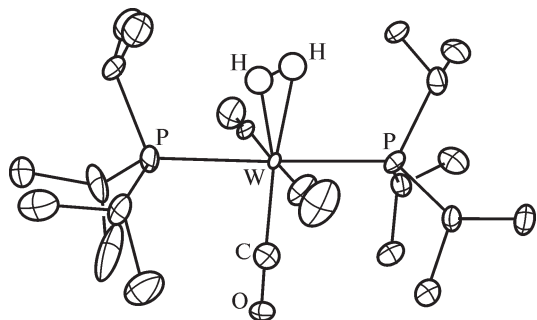
Рис. 3.2. Геометрия ос-транс -[W(CO) 3 (η 2 -H 2 )(PPR 3 i ) 2 ] по данным рентгеноструктурного анализа и нейтронографии: r(\text{H}-\text{H}) = 0,084 нм (ср. с 0,07414 нм для свободной молекулы H 2 ), r(\text{W}-\text{H}) = 0,175 нм. Колебательная ИК-спектроскопия дает \nu(\text{H}-\text{H}) = 2690 см -1 по сравнению с 4159 см -1 для свободной молекулы H 2 (по данным спектроскопии КР)
