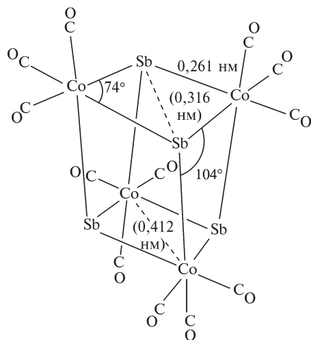
Рис. 13.24. Структура кубаноподобного смешанного кластерного комплекса [Sb_4\{Co(CO)_3\}_4]
