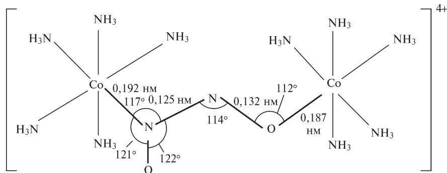
Рис. 11.15. Строение биядерного катиона в красном изомере [\{\text{Co}(\text{NH}_3)_5\text{NO}\}_2](\text{Br})_{2,5}(\text{NO}_3)_{1,5} \cdot 2\text{H}_2\text{O} (средняя длина связи \text{Co}-\text{NH}_3 0,194 \pm 0,002 нм, средний угол 90 \pm 4^\circ )
