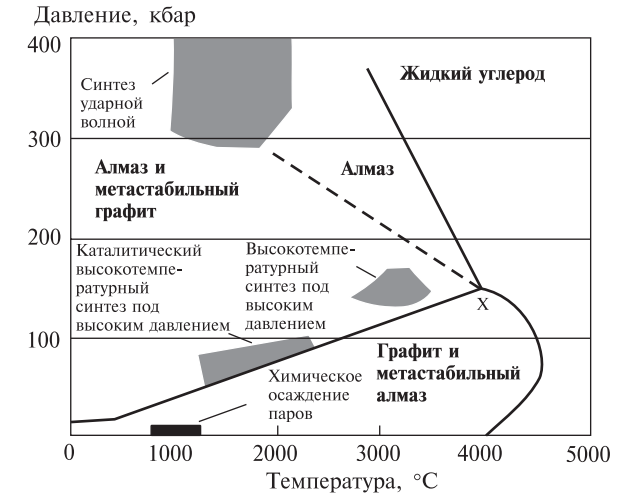
Рис. 8.4. Фазовая диаграмма углерода; показаны области температуры и давления, наиболее важные для получения синтетических алмазов [13]
