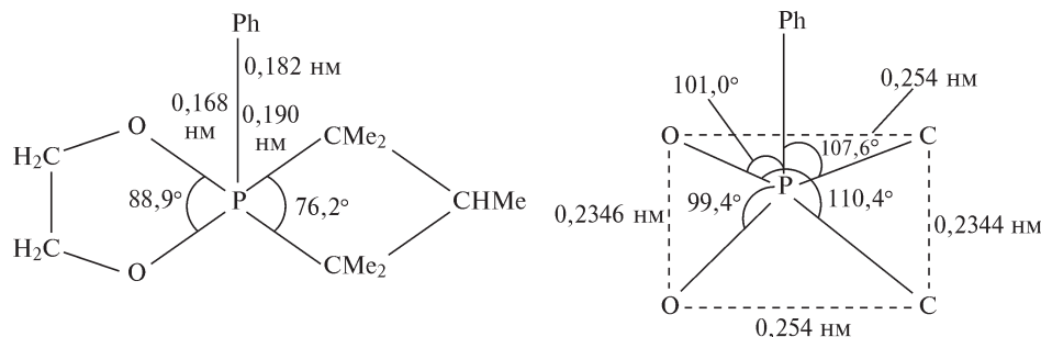
Рис. 12.31. Схематическое изображение строения молекулы [P(C_3H_5Me)(O_2C_2H_4)Ph] ; показано пирамидальное (пирамида с прямоугольным основанием) расположение пяти атомов, связанных с P; атом P находится на расстоянии 0,044 нм над плоскостью C_2O_2
