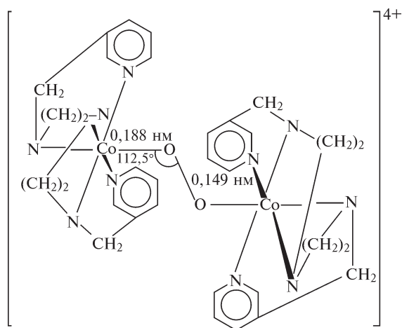
Рис. 14.7. Схематическое изображение строения двухядерного катиона в [\{\text{Co}(\text{pydien})_2\text{O}_2\}]_4^{4+}
