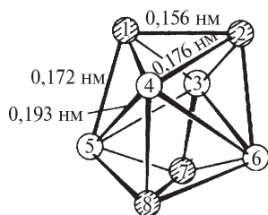
(3) Конфигурация D_{2d} атомов бора в B_8H_8^{2-} ; показаны два структурно неэквивалентных набора из 4 атомов бора
