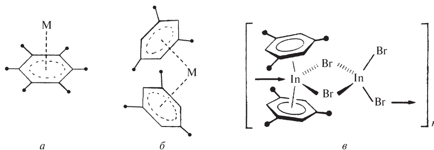
Рис. 7.21. «Полусэндвичевая» структура ( C_{6v} ), характерная для Ga(\eta^6-C_6Me_6)]^+ (а). «Скошенная сэндвичевая» структура, найденная в ионах типа [In(\eta^6-C_6Me_6)_2]^+ (б). Фрагмент спиральной цепи в [In(\eta^6-mes)_2][InBr_4] (в); показана мостиковая группировка [\mu-\eta^1, \eta^2-InBr_4] между ионами, изображенными на рис. (б). Угол равен 133^\circ , а центры двух ареновых лигандов почти равноудалены от атома индия (0,283 и 0,289 нм)
