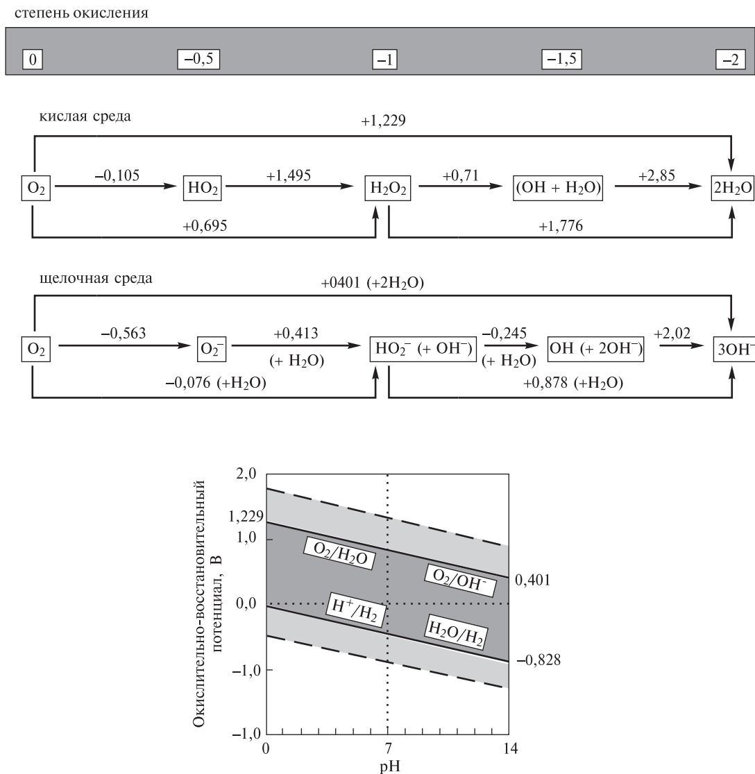
Рис. 14.12. Изменение окислительно-восстановительных потенциалов пар \text{O}_2/\text{H}_2\text{O} и \text{H}^+/\text{H}_2 (или \text{O}_2/\text{OH}^- и \text{H}_2\text{O}/\text{H}_2 ) в зависимости от pH (сплошные линии). Штриховые линии, лежащие на 0,5 В выше и ниже сплошных линий, показывают приблизительные практические пределы значений потенциалов для окислителей и восстановителей в водных растворах, когда сам растворитель окисляется до \text{O}_2(\text{г}) или восстанавливается до \text{H}_2(\text{г})
