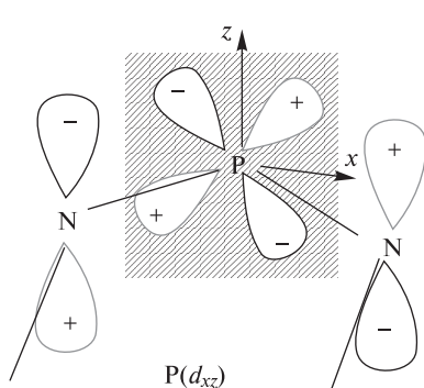
в Изображение в перспективе возможного \pi -связывания (гетероморфное p\pi-d\pi -взаимодействие между Np_z и P(d_{xz}) ), а также возможные гомоморфные p\pi-d\pi -взаимодействия орбиталей Np_z через орбиталь P(d_{xz}) .
