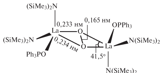
Рис. 14.8. Строение плоского центрального фрагмента мостикового пероксокомплекса [\text{La}\{\text{N}(\text{SiMe}_3)_2\}_2(\text{OPPh}_3)]_2\text{O}_2
