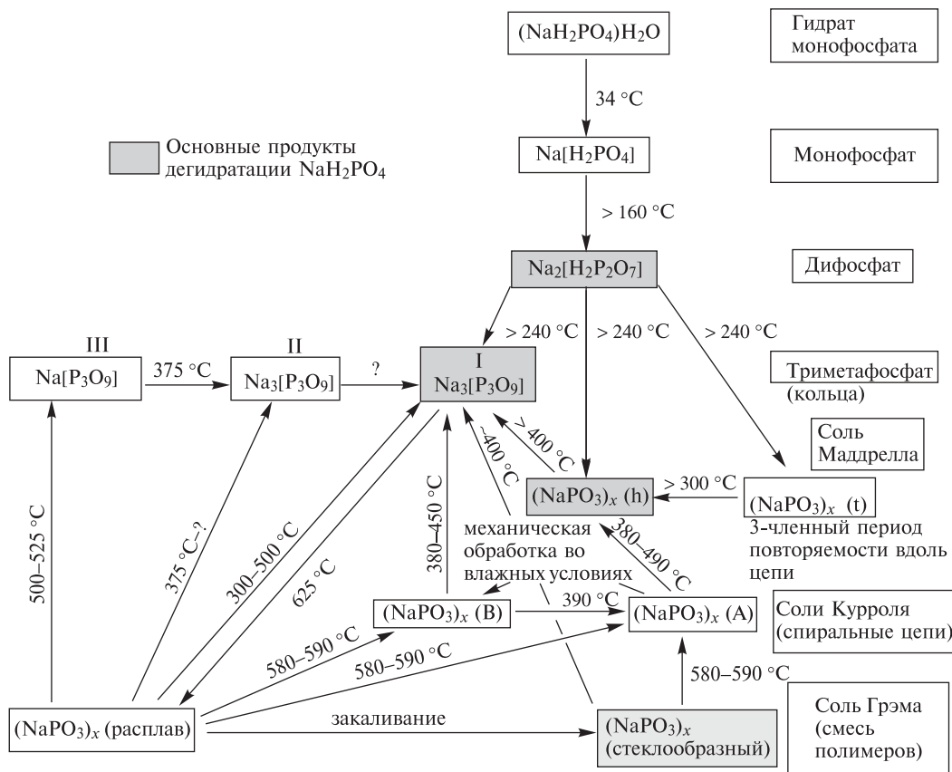
Рис. 12.21. Взаимопревращения метафосфатов [CIC, Vol. 2, p. 521]
