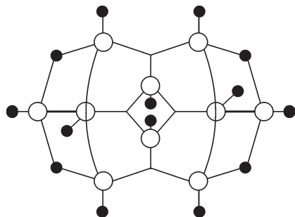
B_{10}H_{14} (4620)
