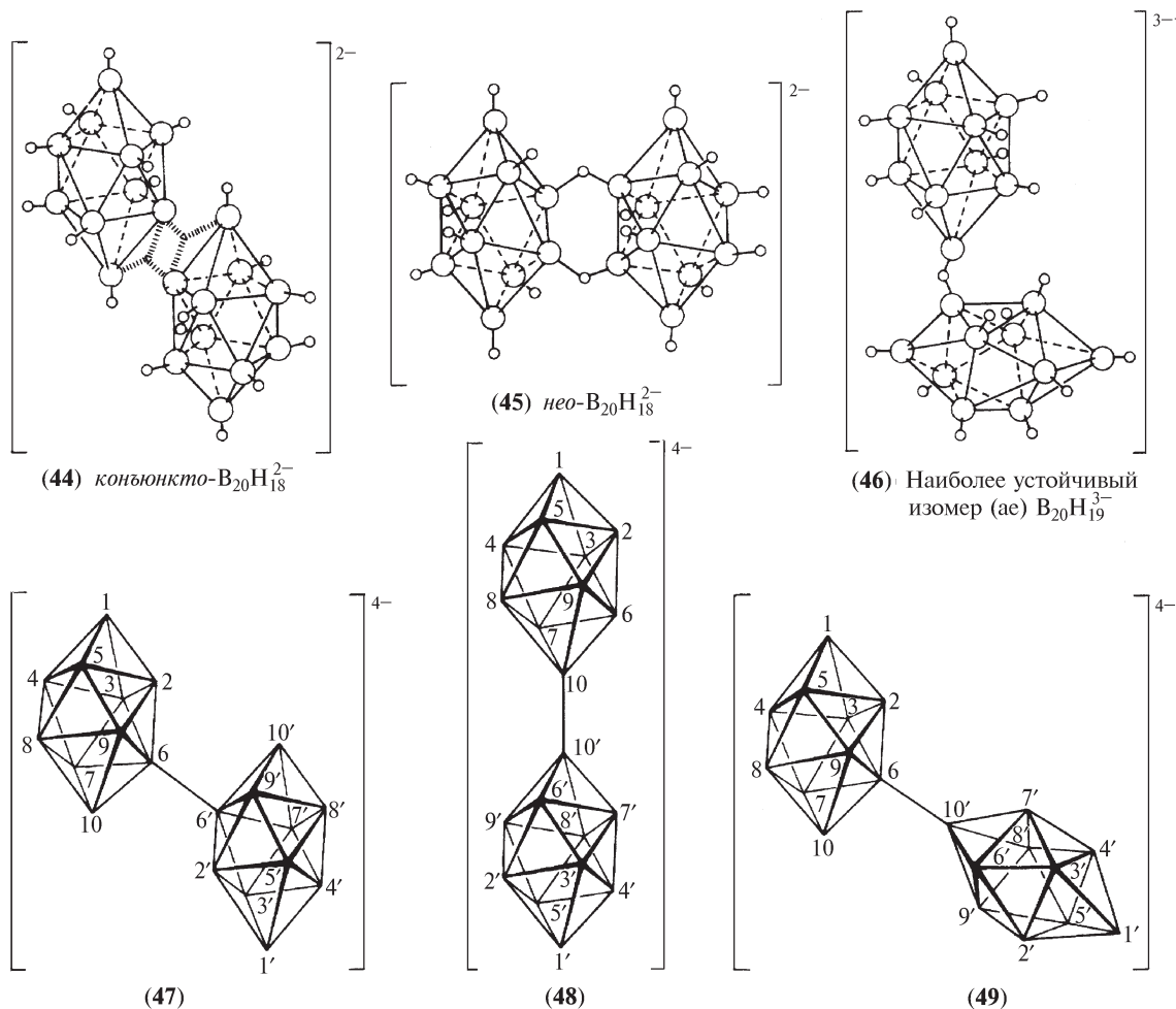
Структуры трех изомеров конъюнкто- B_{20}H_{18}^{4-}
