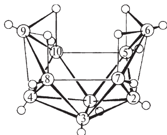
(11) B_{10}H_{14}
