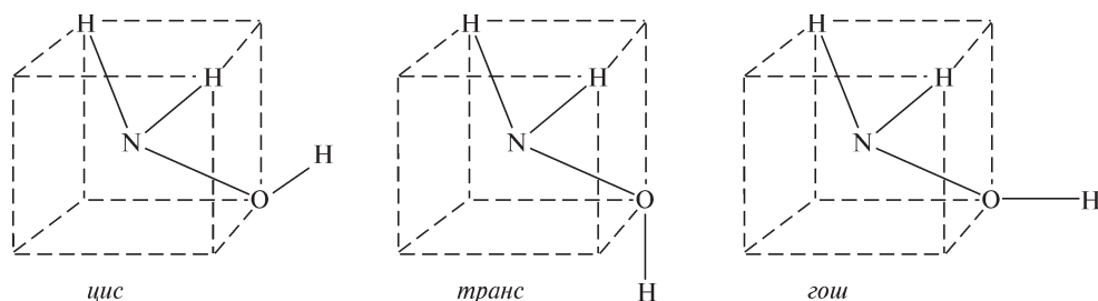
Рис. 11.7. Конфигурации \text{NH}_2\text{OH}
