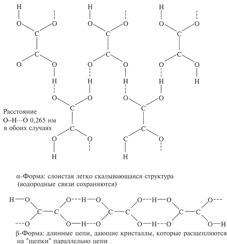
Рис. 3.9. Схематическое изображение двух форм щавелевой кислоты (—CO 2 H) 2
