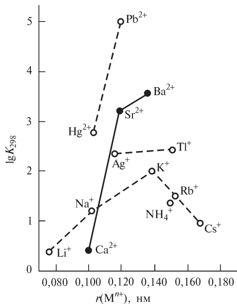
Рис. 5.6. Константы образования K для комплексов полиэфира дициклогексано-18-краун-6 с различными катионами. Следует отметить, что, хотя радиусы \text{Ca}^{2+} , \text{Na}^+ и \text{Hg}^{2+} очень близки, соотношение констант образования составляет 1 : 6,6 : 225. Для \text{K}^+ и \text{Ba}^{2+} , которые также имеют близкие радиусы, соотношение констант равно 1 : 35 (шкала логарифмическая)
