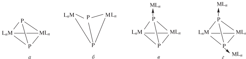
Рис. 12.7. a — (\mu, \eta^2-P_2) как 4-электронный донор по отношению к 15-электронным вершинам ML_n ; б — (\mu, \eta^2-P_2) как 4-электронный донор по отношению к 14- или 16-электронным ML_n ; в — тройной мостик (\mu_3, \eta^2-P_2) , формально 6-электронный донор; г — четверной мостик (\mu_4, \eta^2-P_2) , 8-электронный донор
