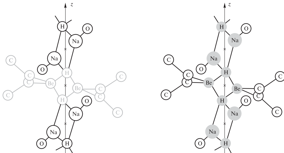
Рис. 5.9. Кристаллическая структура эфирата полимерного гидриодиэтилбериллата натрия [\text{Et}_2\text{ONaHBeEt}_2]_n (выделены две особенности структуры (см. текст)).
