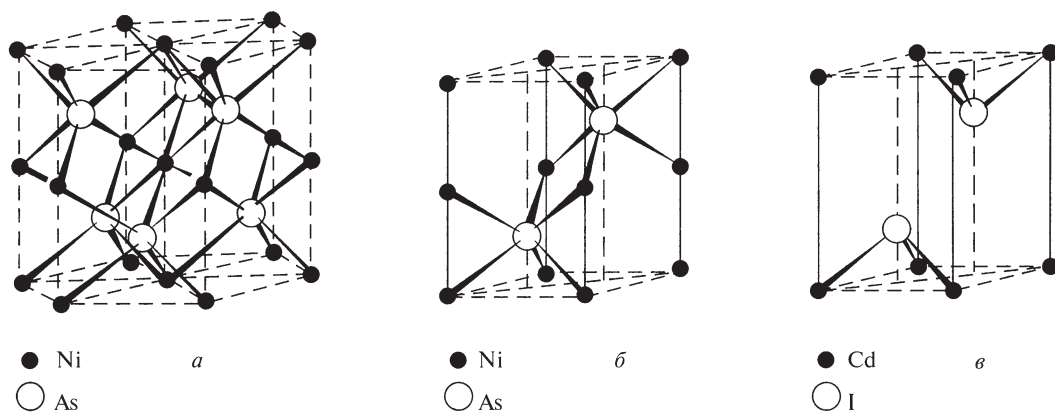
Рис. 13.3. Структура арсенида никеля: a — три элементарные ячейки; b — одна элементарная ячейка ( \text{Ni}_2\text{As}_2 ); в — элементарная ячейка слоистой структуры \text{CdI}_2 (для сравнения, см. текст)
